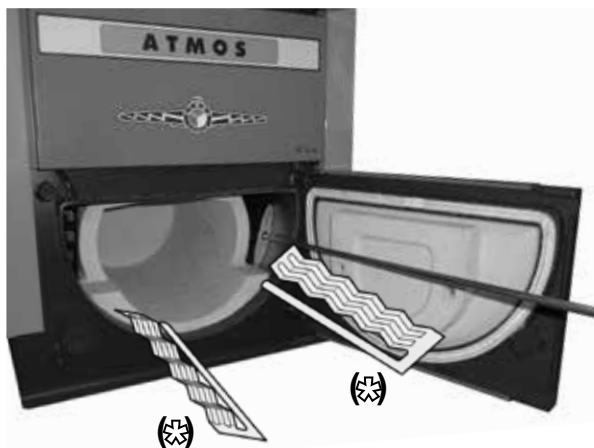
Offene untere Tür mit der Keramik-Kuglarum ausgestattet und seine Reimigung-Seitenwände der Verbrennungskammer durch den Putzschaber *Nur bei DC22GSE und DC30GSE
